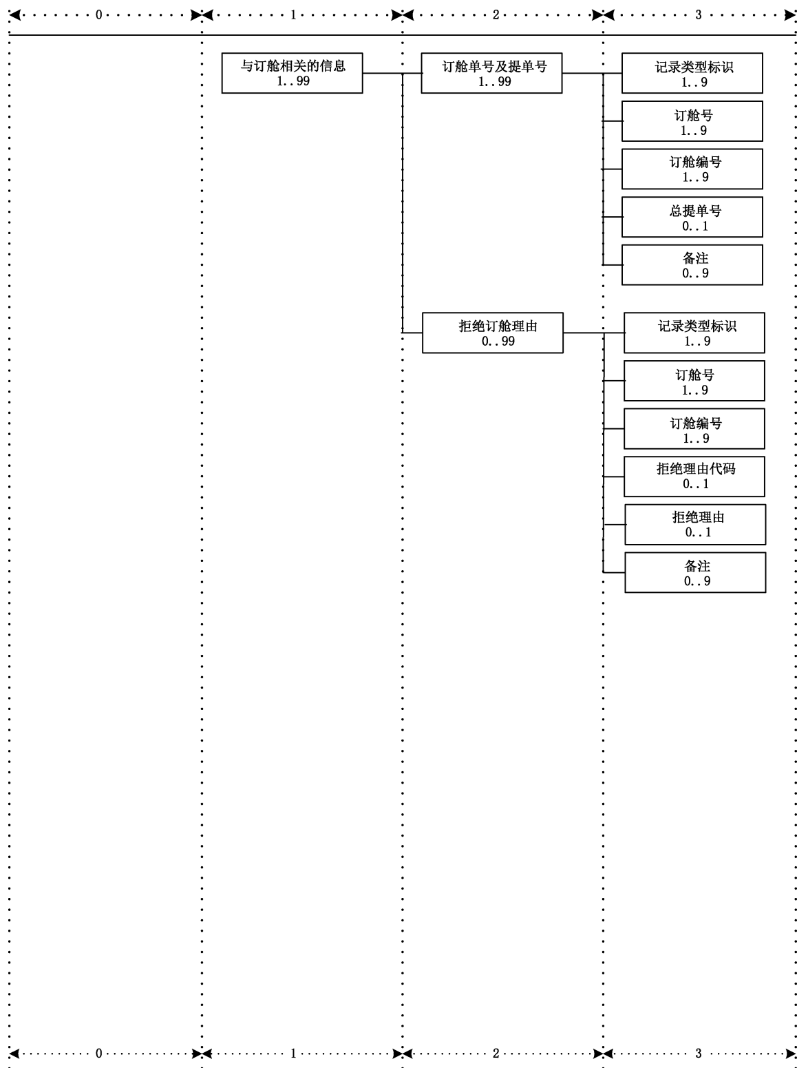
图 3 描述订舱单号及提单号/拒绝订舱理由结构
